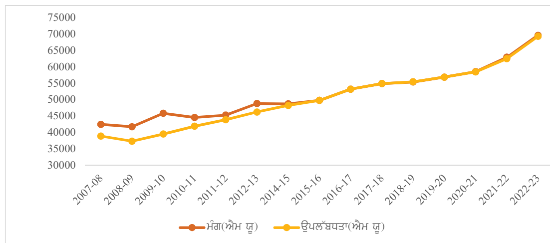
ਚਿੱਤਰ 53: ਪੰਜਾਬ ਵਿਚ ਬਿਜਲੀ ਦੀ ਮੰਗ ਅਤੇ ਉਪਲੱਬਧਤਾ
